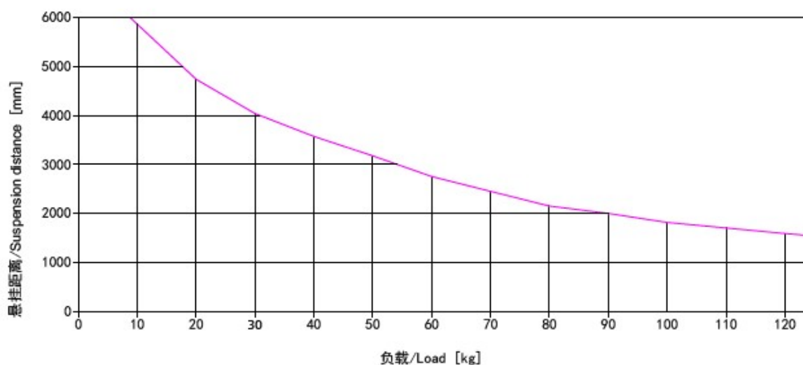
承载力数据图 A065 (仅供参考) / Load chart profile A065 (For reference only)
