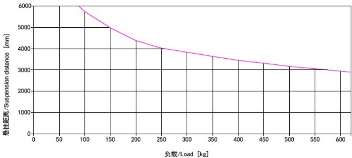
承载力数据图 AM（仅供参考） / Load chart profile AM（For reference only）
