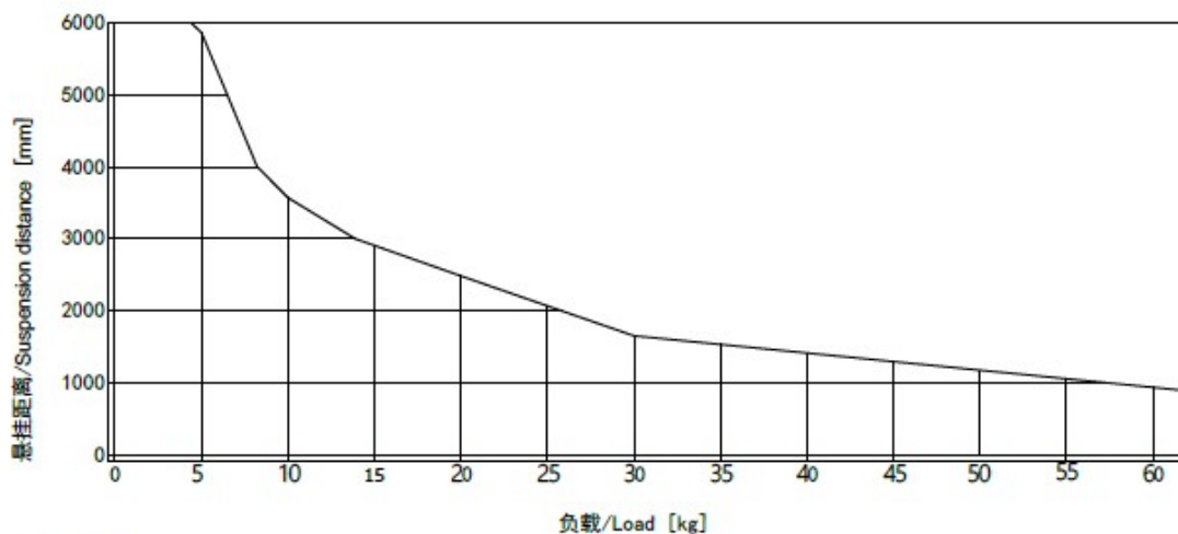
承载力数据图 A055 (仅供参考) / Load chart profile A055 (For reference only)
