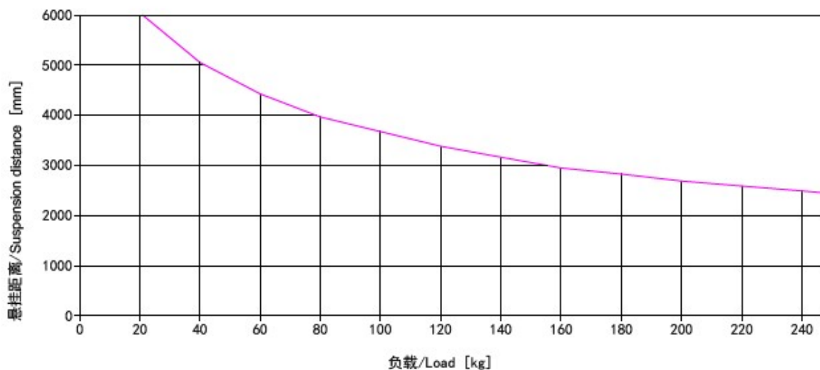
承载力数据图 A105（仅供参考） / Load chart profile A105（For reference only）
