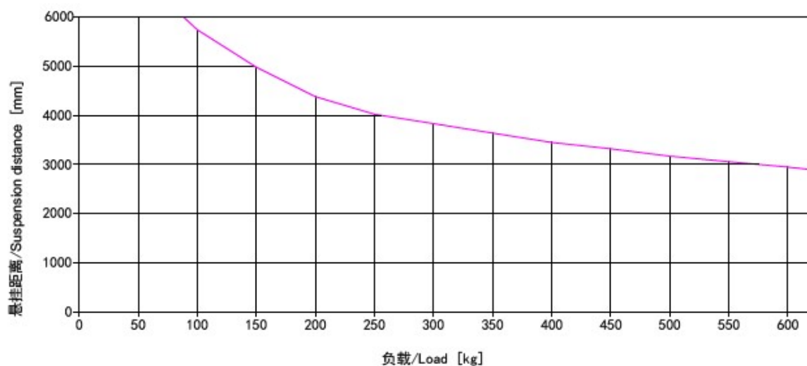
承载力数据图 A140（仅供参考） / Load chart profile A140（For reference only）
